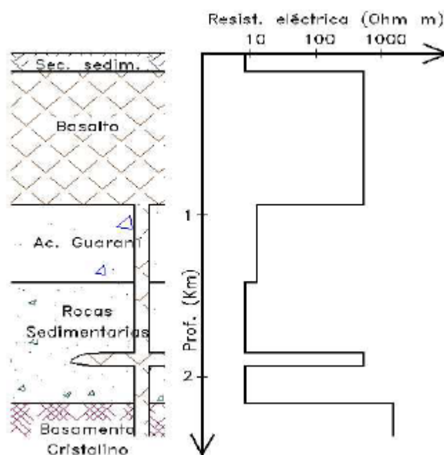
Figura 13. Corte litológico en el área de estudio con el registro eléctrico correspondiente (Oleaga, 2002).
