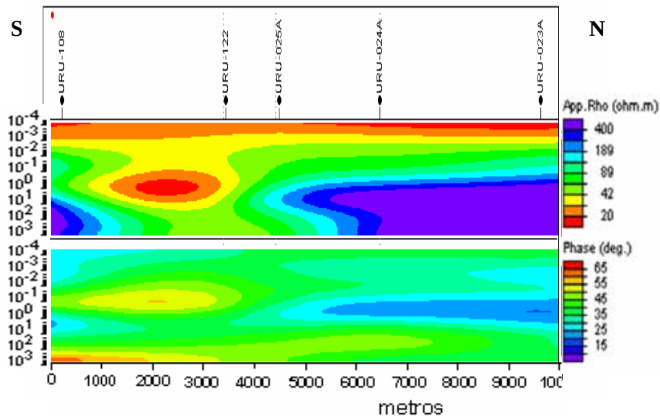
Figura 36. Perfil 1, modo TE
