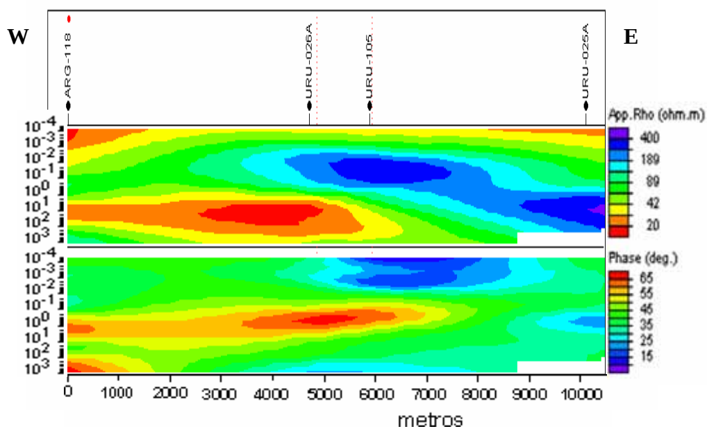
Figura 54. Perfil 10, modo TE
