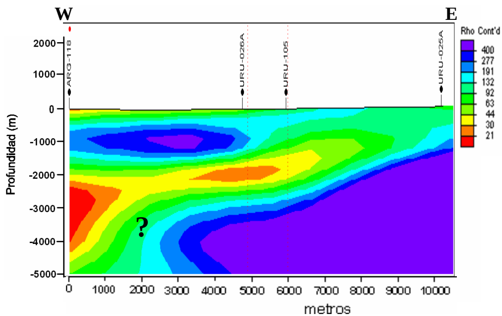
Figura 75. Perfil 10. Interpolación 1D
