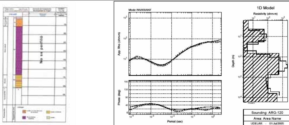
Figura 63. Paramétrico pozo Chajari, Sondeo 120
