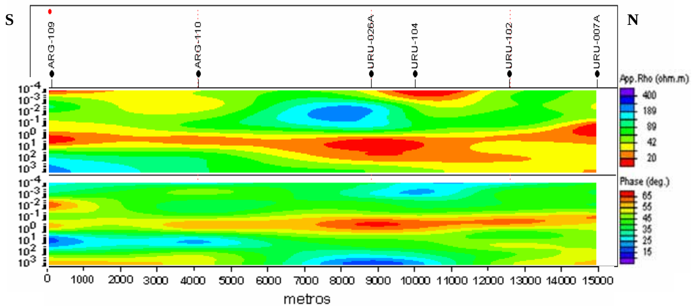
Figura 40. Perfil 3, modo TE
