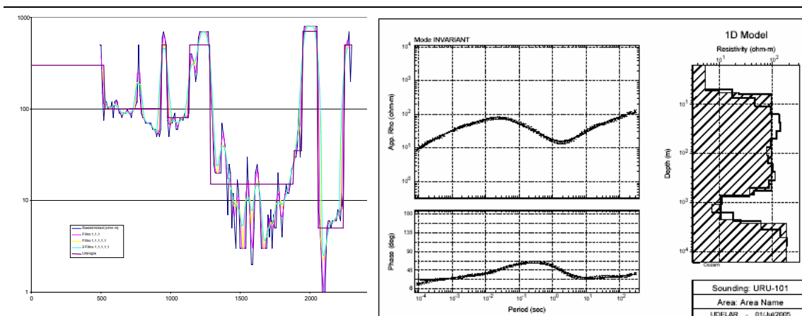
Figura 58. Paramétrico pozo Gaspar, Sondeo 101
