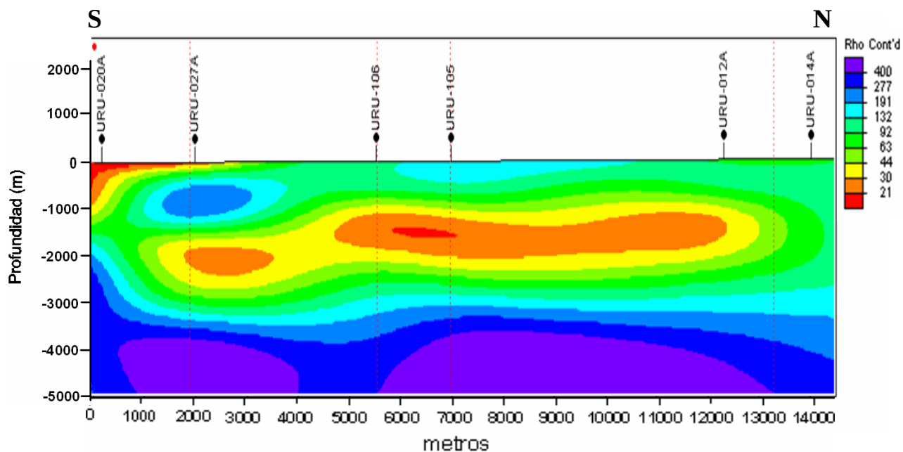
Figura 69. Perfil 2. Interpolación 1D
