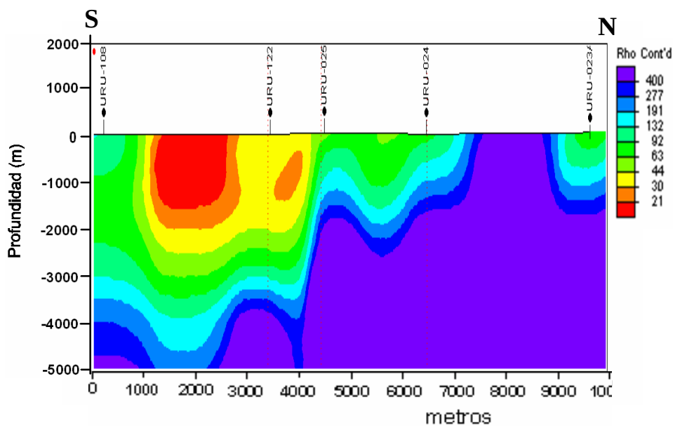
Figura 84. Perfil 1, análisis 2D
