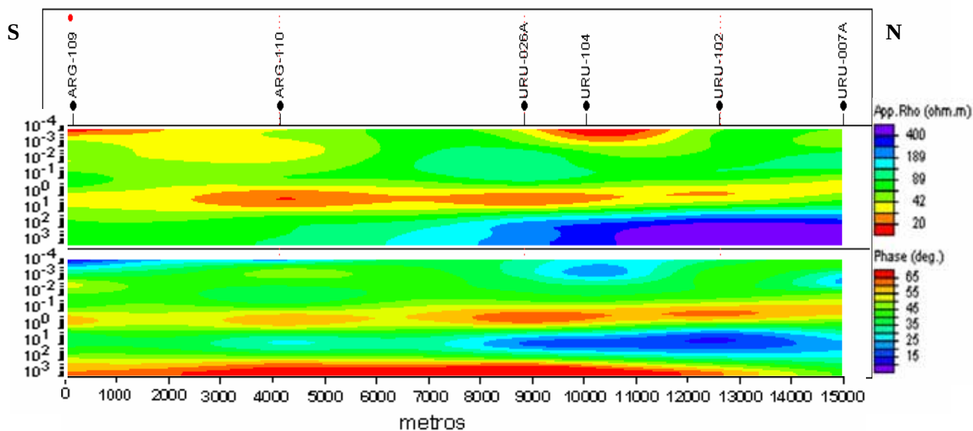
Figura 41. Perfil 3, modo TM
