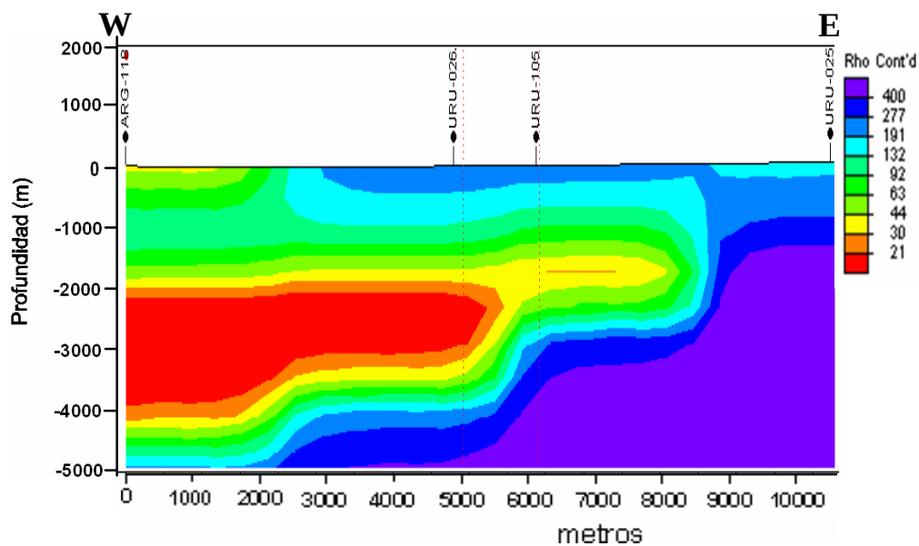
Figura 91. Perfil 10, análisis 2D
