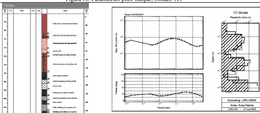
Figura 59. Paramétrico pozo Belén, Sondeo 5
