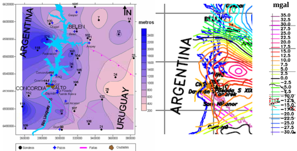
Figura 81. Izquierda espesor de basaltos, derecha anomalía de Bouguer (Subiza et al., 1994)
